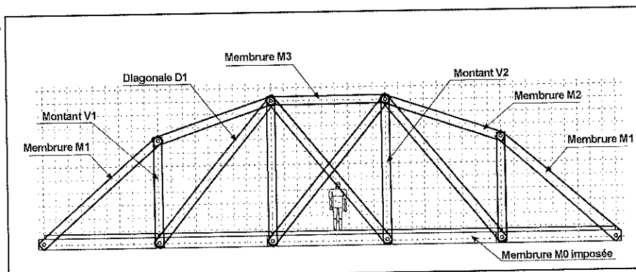
Exemple de dessin finalisé
